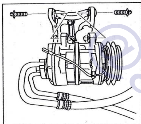
شکل ۶-۳-۱۰: پیاده سازی کمپرسور A/C
