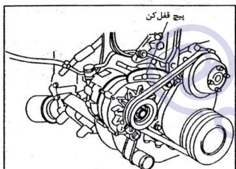
شکل ۱۰-۳-۱۰: نصب آلترناتور
