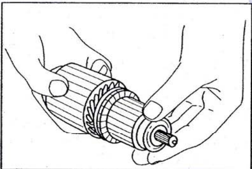
شکل ۲۸-۲-۱۰: بررسی بلبرینگ
