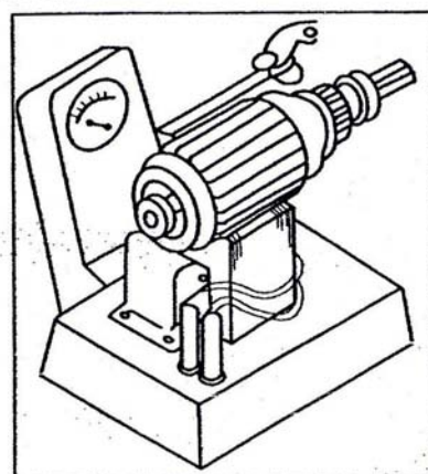
شکل ۱۰-۲-۲۰: تست اتصال کوتاه آرمیچر
