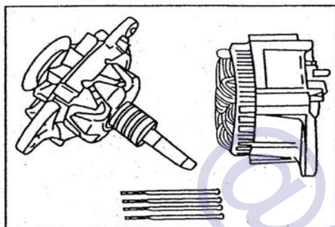
شکل ۱۰-۳-۱۹: پیاده سازی دینام
