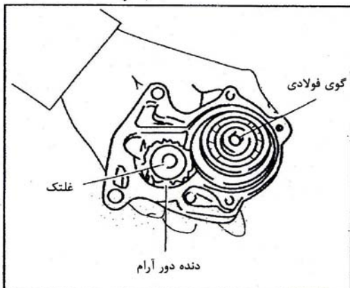
شکل ۲۹-۲-۱۰: نصب دنده دور آرام و غلاف
