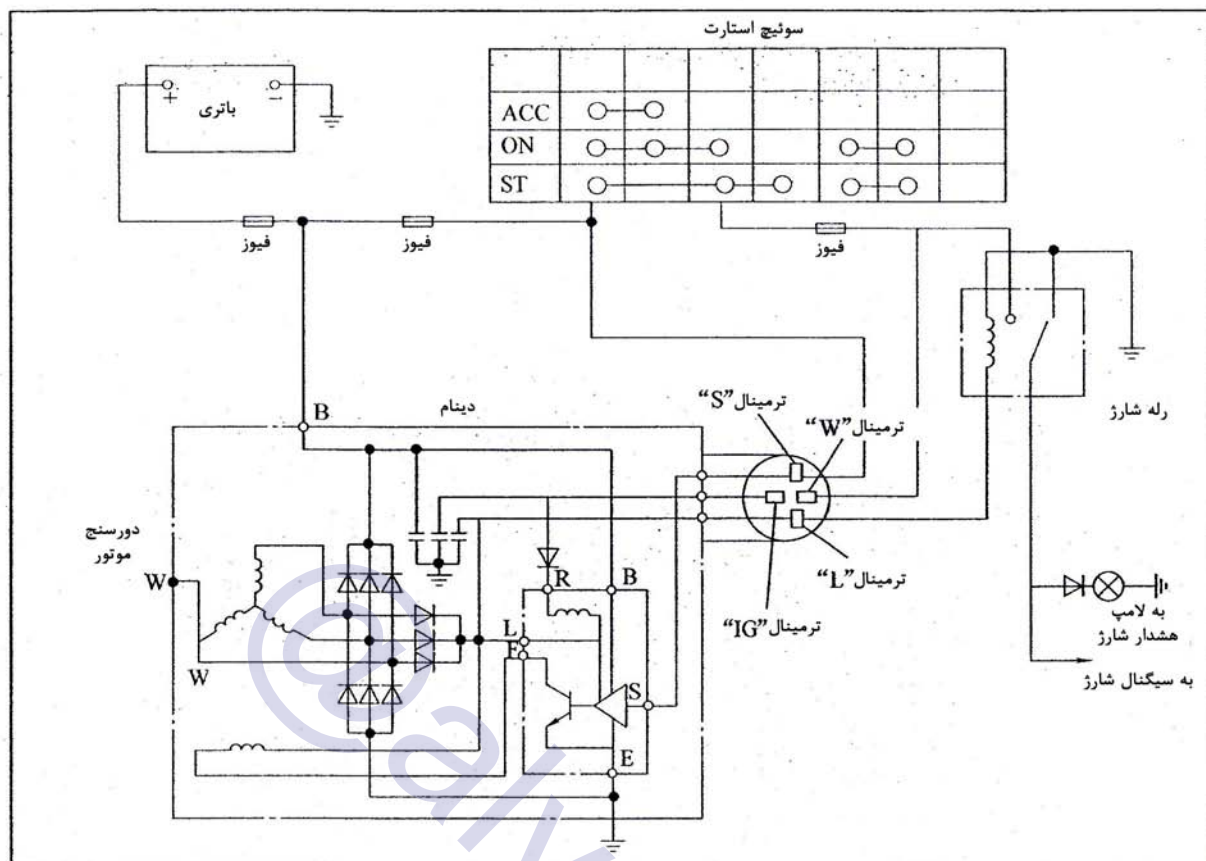
شکل ۱۰-۳-۲: مدار شارژ
