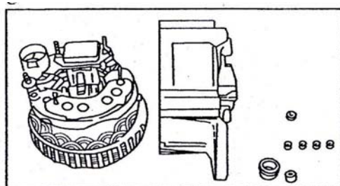
شکل ۱۰-۳-۲۱: پیاده سازی دینام
