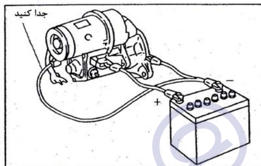
شکل ۱۰-۲-۳۱: تست نگهداری
