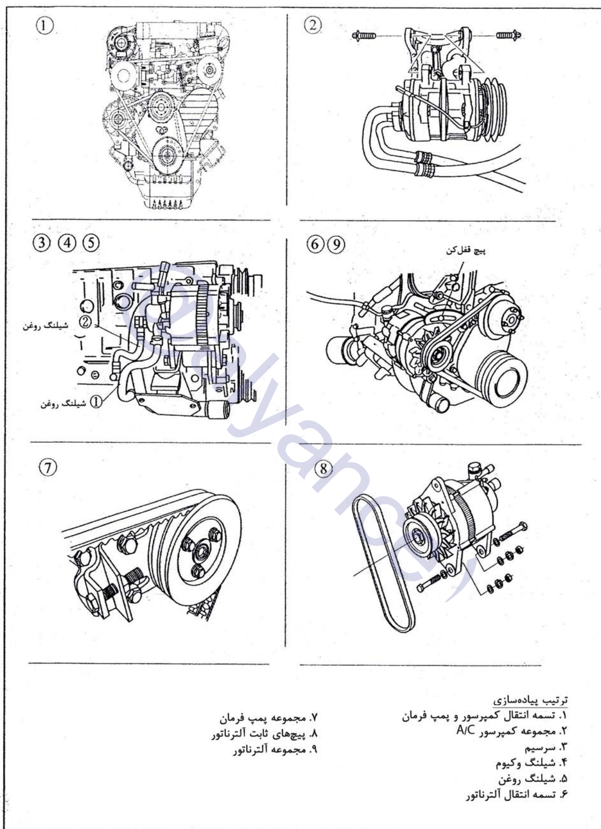
شکل ۳-۱۰: ترتیب باز و بسته کردن موتور
