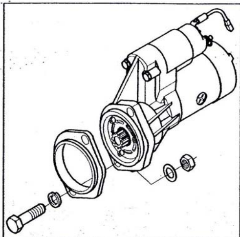
شکل ۱۰-۲-۵: پیاپی سازی مجموعه استارت
