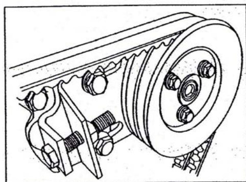
شکل ۸-۳-۱۰: پیاده سازی مجموعه پمپ فرمان
