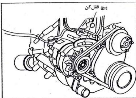
شکل ۷-۳-۱۰: پیاده سازی تسمه انتقال آلترناتور
