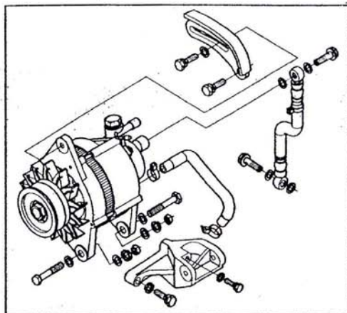
شکل ۹-۳-۱۰: پیاپاده‌سازی مجموعه آلترناتور
