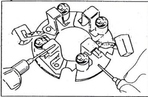
شکل ۲۶-۲-۱۰: تست عایق پایه ذغال
